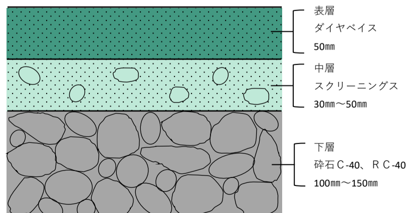
● テニスコートの標準断面図
