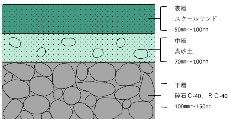
● 学校グラウンドの標準断面図
